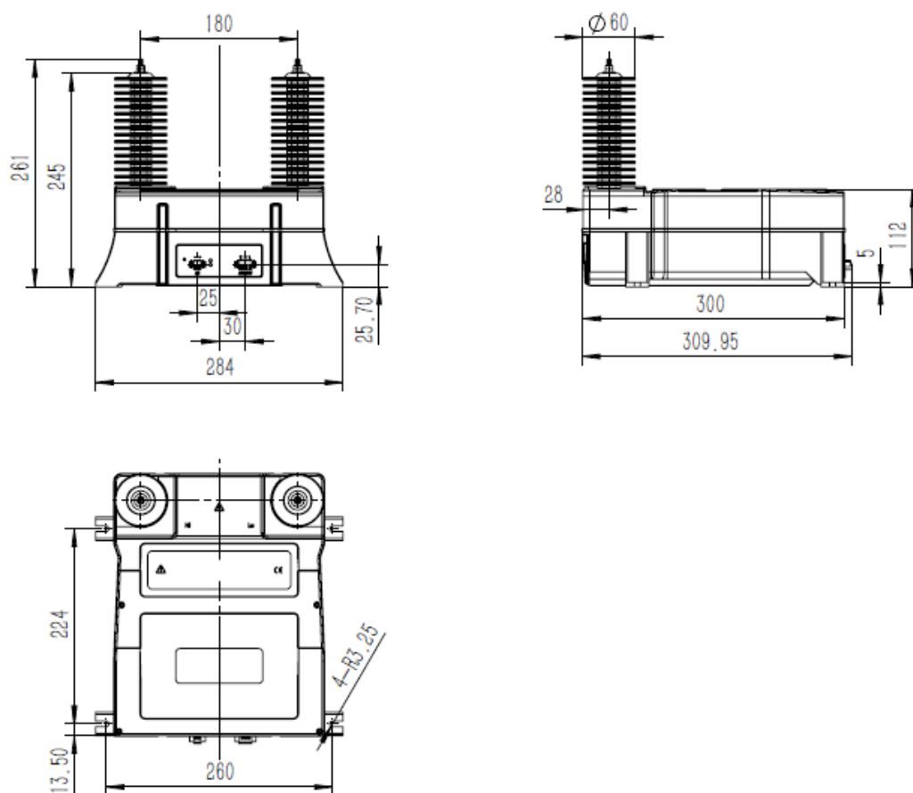
图 1 外形尺寸图
