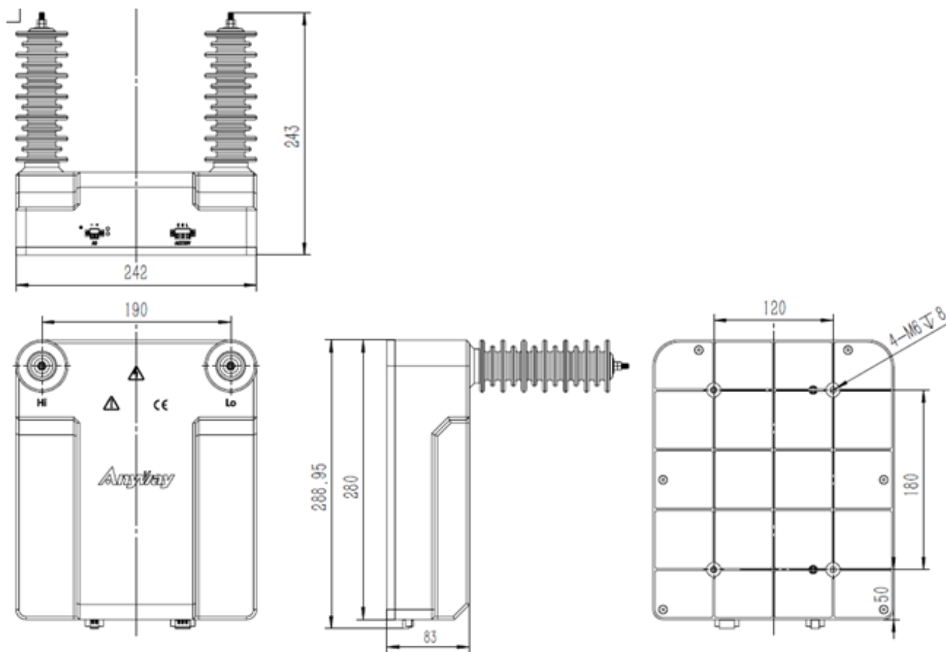
图 1 外形尺寸图
