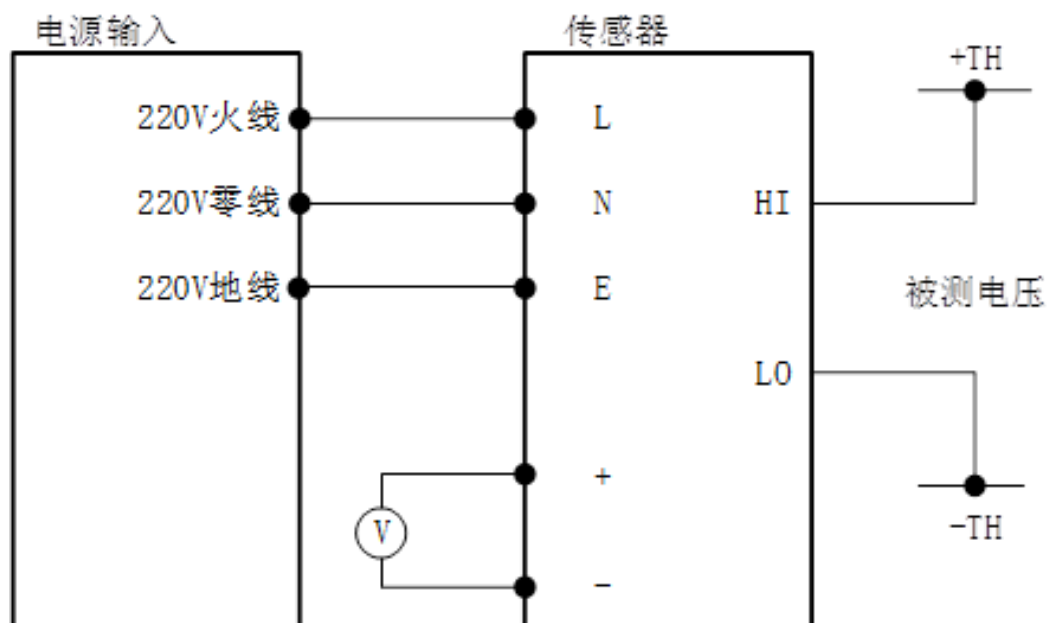
图 3 电气连接图
