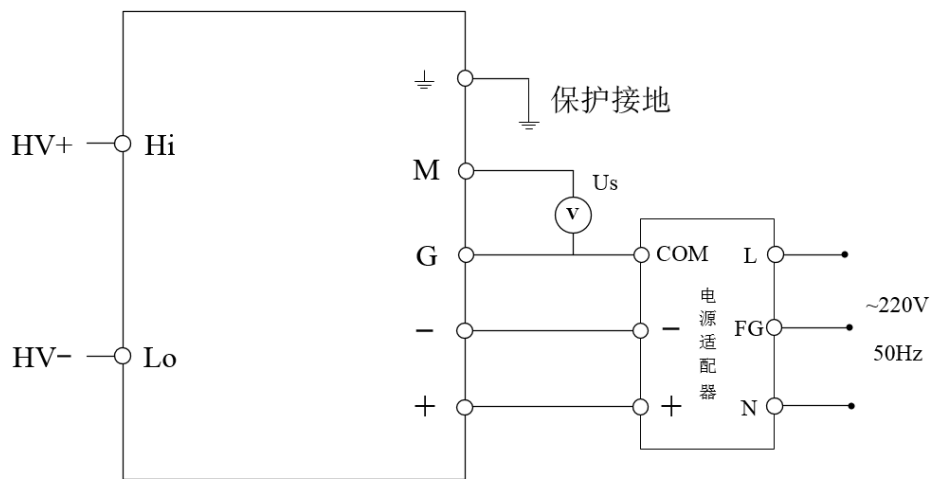
图 3 电气连接图
