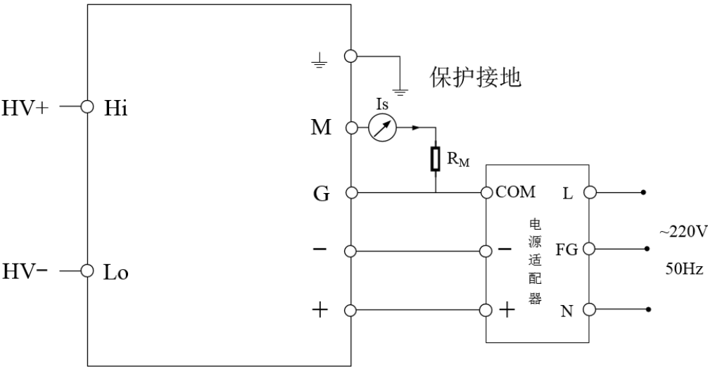
图 3 电气连接图
