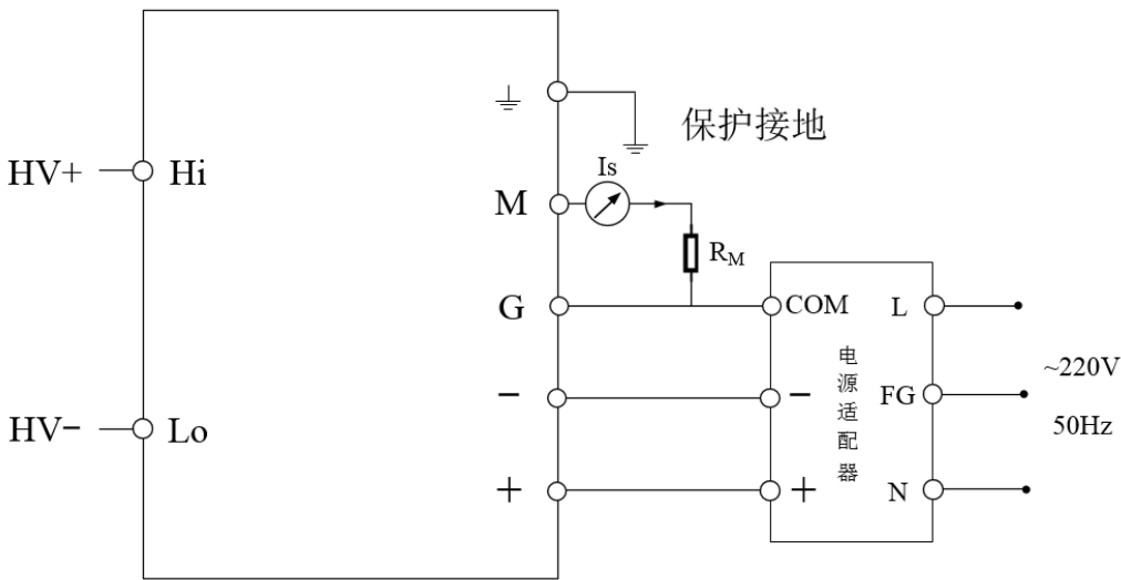
图 3 电气连接图
