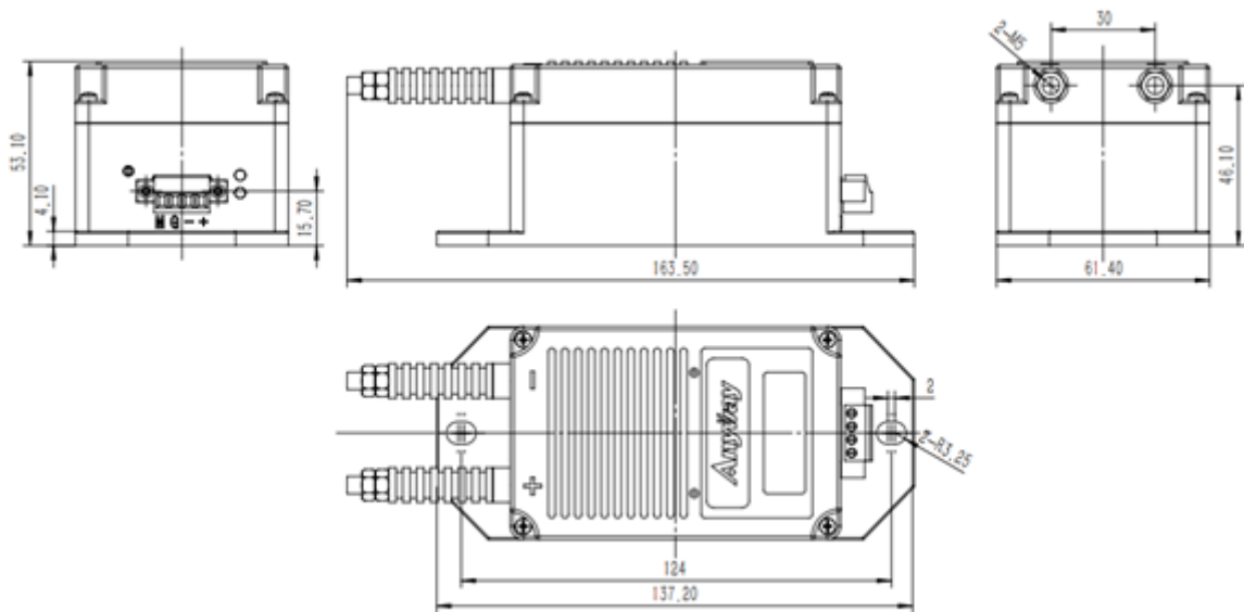
图 1 外形尺寸图
