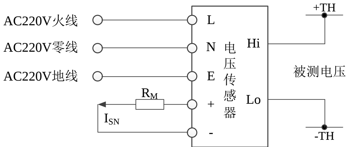
图3 电气连接图
