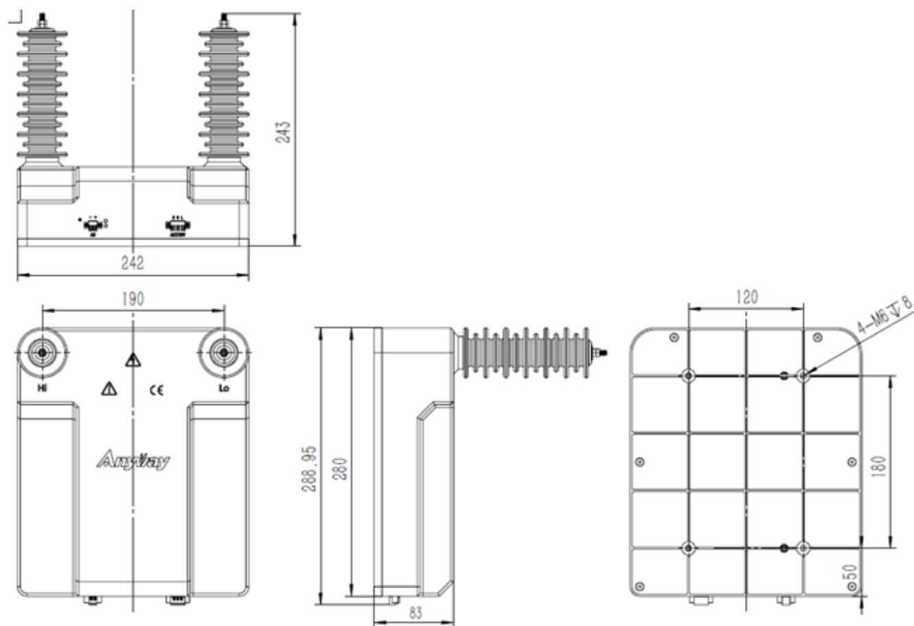
图 1 外形尺寸图
