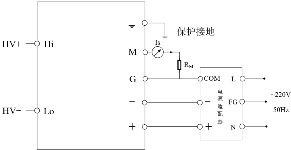
图 3 电气连接图
